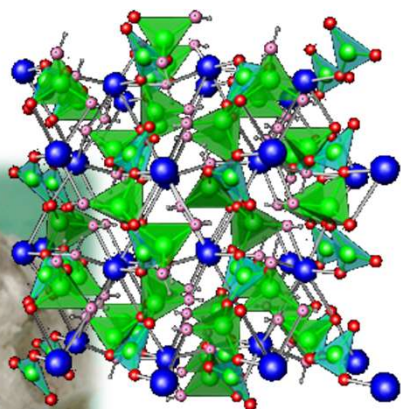
Јарандолит \text{Ca}[\text{B}_3\text{O}_4(\text{OH})_3]
